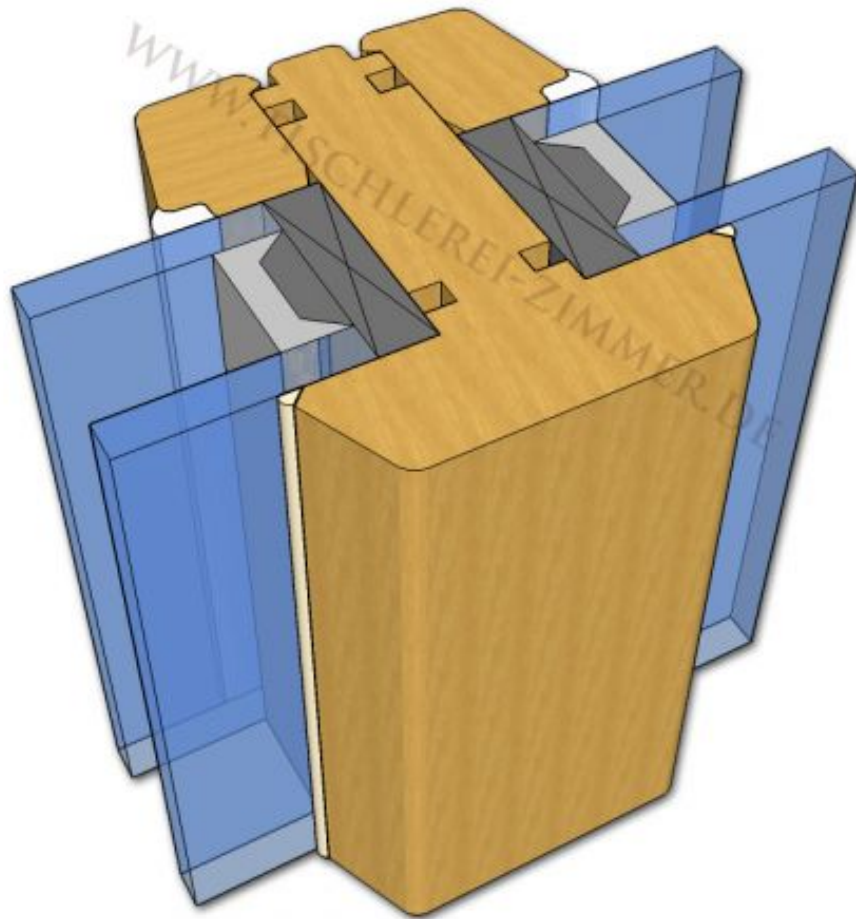
glasteilende Sprosse (standard)
